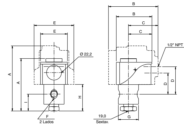
Desenho 1 - Válvula NF, NA e U 1/8" (latão/inox) 1/4" (inox) NPT/BSP
