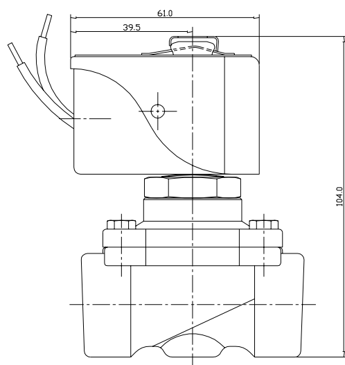
Desenho 1 - Válvula N.F. NPT/BSP
